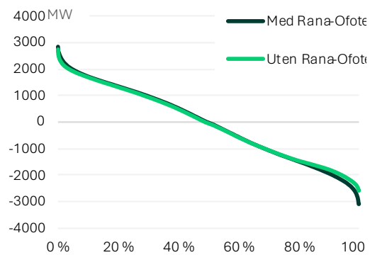
Figur 80: Virkning på flyt på Hålogalandssnittet (ut av Nord-Norge) i 2050 i basis med og uten Rana–Ofoten på 420 kV.
