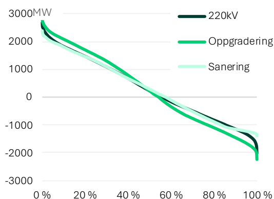
Figur 34: Varighetskurve for flyt over Hålogalandssnittet (ut av Nord-Norge) i 2035 Basis.
