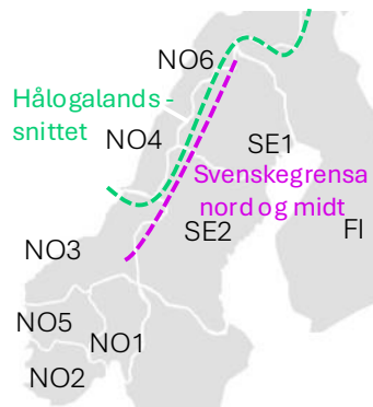
Figur 38: Kart med de sentrale storsnittene
