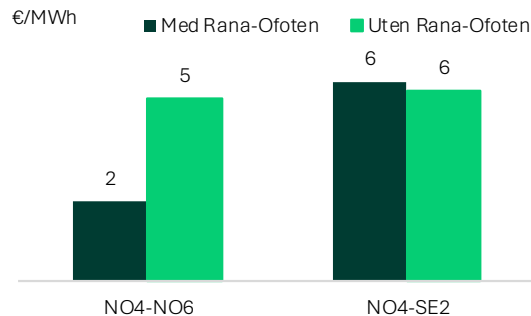
Figur 76: Absolutt gjennomsnittlig prisforskjell i 2050 med Oppgradering, i Basis og uten dublert Rana-Ofoten.
