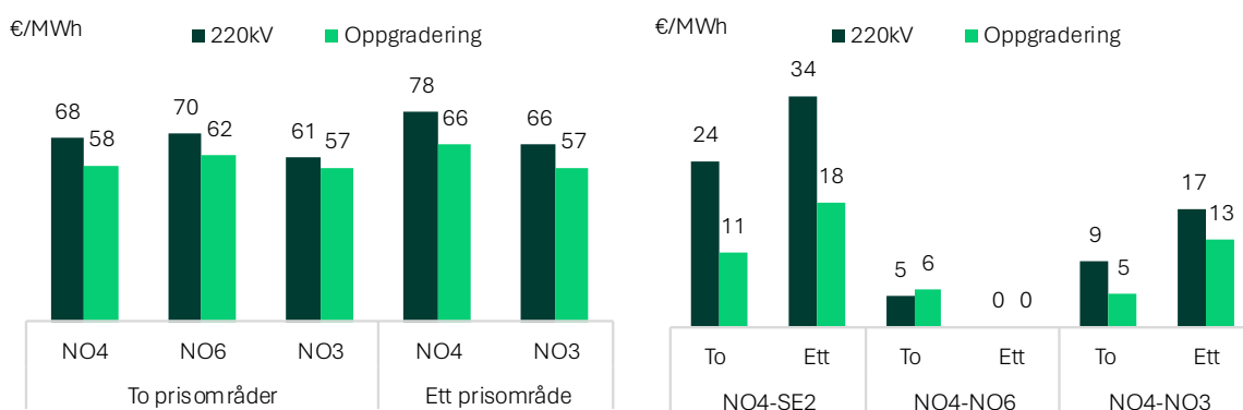
Figur 73: Snittpris i 2035 med underskudd (-4 TWh) på energibalansen i Nord-Norge
