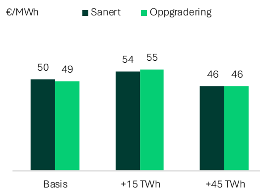
Figur 69: Snittpris for NO4 i 2050 med ulike energibalanser i Nord-Sverige. I Basis 2050 er overskuddet rundt 30 TWh i Nord-Sverige
