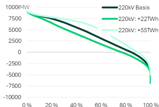
Figur 45: Varighetskurve for flyt mellom SE2 og SE3 i Nullalternativet i 2035 ved ulike energibalanse i Nord-Sverige.
