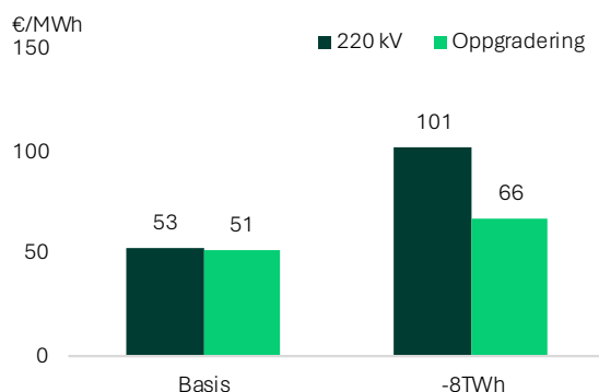
Figur 64: Snittpris i NO4 i 2035 i Basis og med -8 TWh underskudd på energibalansen i Nord-Norge
