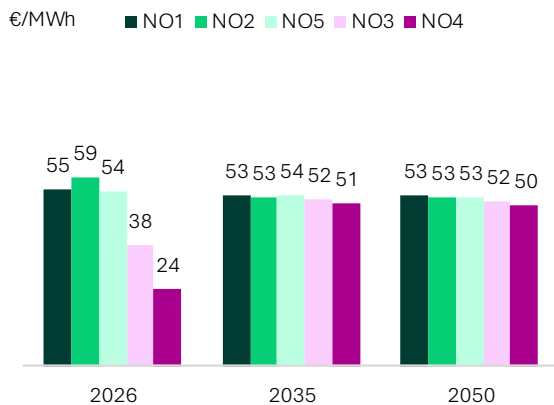
Figur 46: Snittpris i Norge mot 2050
