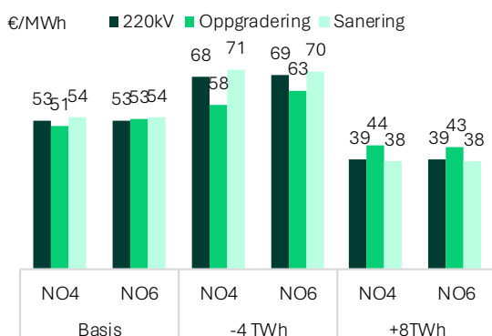
Figur 58: Snittpris i NO4 i 2035 ved underskudd på 4 TWh og overskudd på 8 TWh i Nord-Norge
