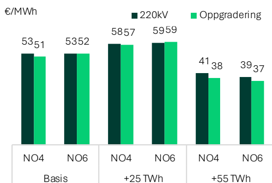
Figur 68: Snittpris for NO4 i 2035 med ulike energibalanser i Nord-Sverige. I Basis 2035 er overskuddet rundt 40 TWh i Nord-Sverige
