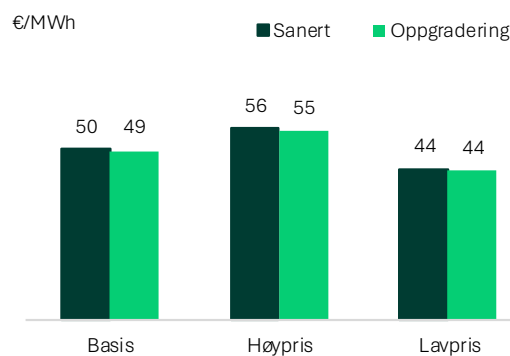
Figur 67: Snittpris i NO4 i 2050 for de ulike konseptene med Høypris og Lavpris
