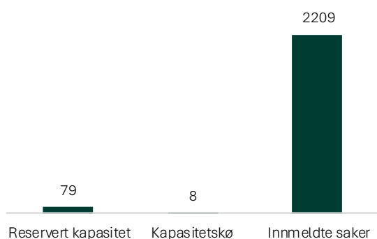
Figur 18: Produksjonsplaner på Helgeland i MW.
