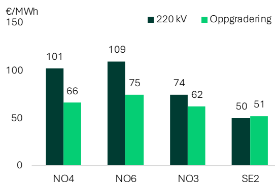
Figur 65: Snittpriser i 2035 med -8 TWh underskudd på energibalansen i Nord-Norge
