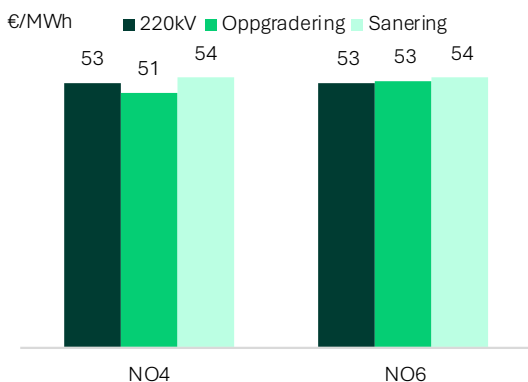
Figur 48: Snittpris for NO4 og NO6 i Basis 2035 (2 TWh overskudd i Nord-Norge)
