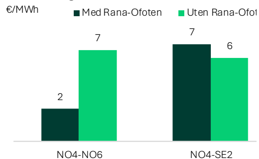
Figur 78: Absolutt gjennomsnittlig prisforskjell i 2050 med -6 TWh underskudd i Nord-Norge.
