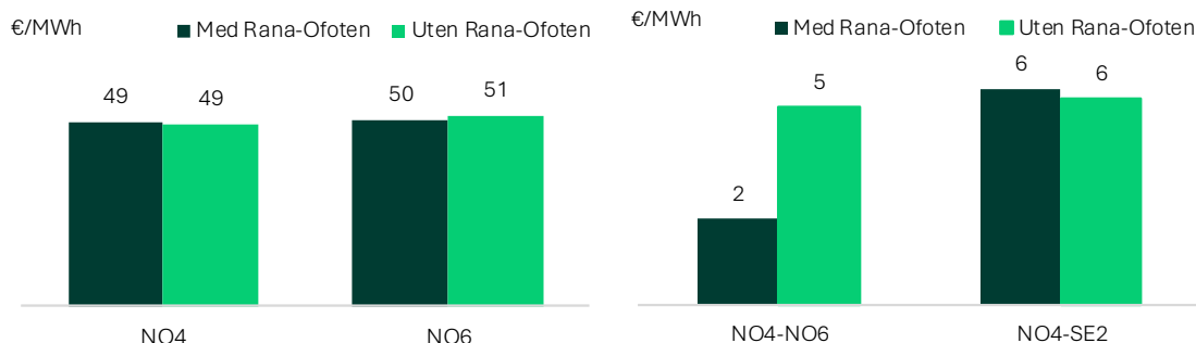
Figur 75: Snittpriser i 2050 med Oppgradering, i Basis og uten dublert 420 kV Rana-Ofoten.
