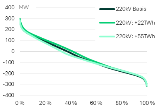
Figur 44: Varighetskurve for flyt mellom NO4 og SE2 i Nullalternativet for 2035 ved ulike energibalanse i Nord-Sverige.
