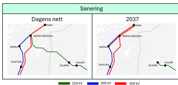
Figur 24: Illustrasjon av saneringskonseptet
