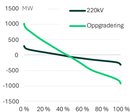
Figur 29: Varighetskurve for flyt NO4–SE2 i 2035 Basis.
