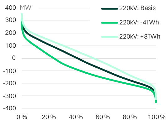
Figur 42: Varighetskurve for kraftflyt mellom NO4–SE2 i Nullalternativet for 2035 ved ulike energibalansen i Nord-Norge.
