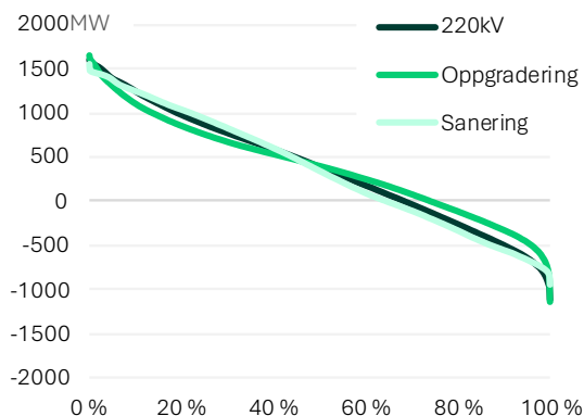
Figur 36: Varighetskurve for flyt mellom NO3 og NO4 i 2035 Basis.
