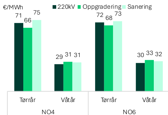
Figur 50: Snittpris i NO4 og NO6 i 2035 Basis i et tørrår og et våtår.
