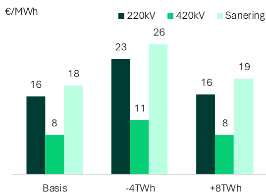
Figur 62: Absolutt gjennomsnittlig prisforskjell mellom NO4–SE2 i 2035 med ulike energibalansen
