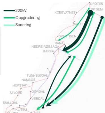
Figur 31: Kart med de mest begrensende snittene i hvert konsept i 2035-nettet 13
