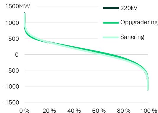
Figur 37: Varighetskurve for flyt mellom NO4–NO6 (Svartisen–Salten) i 2035 Basis.
